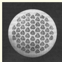
Bi2212線材 (2mm径) 1320芯 臨界電流1000A (4K) 超強磁場用 (日立製作所)
