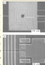
金属超伝導 dc SQUID Nb/Al ジョセフソン接合
