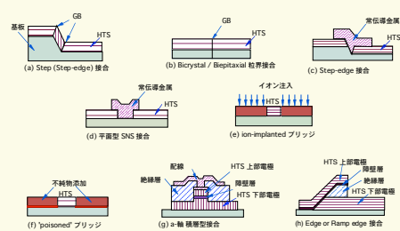
高温超伝導体のジョセフソン接合構造
