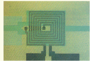
高温超伝導 dc SQUID YBCO bieptaxial 粒界ジョセフソン接合
