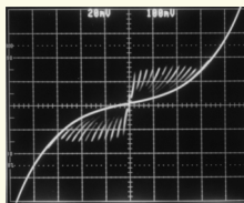
Bi 2 Sr 2 CaCu 2 O 8+δ 微小メサ素子の電流電圧特性
